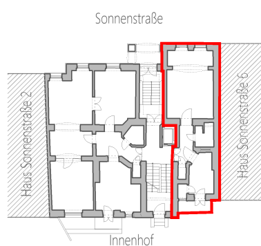
Übersicht EG
